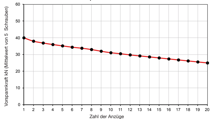
Vorspannkraftverlauf
